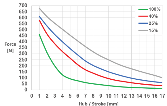
Kraft / Weg-Kennlinie Kühlblech
